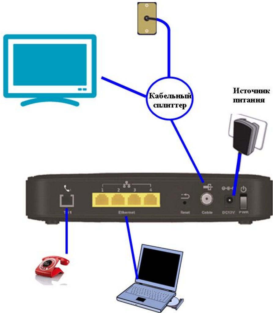
Рис. 1 «Экран коаксиального кабеля необходимо подключить с заземлением».
